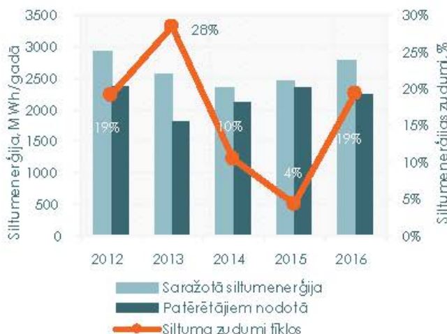
2.8. ATTĒLS: Saražotā un patērētājiem nodotie siltumenerģijas apjomi un siltumenerģijas zudumi katlu mājā Pilsrundālē (augšā) un Saulainē (apakšā).
