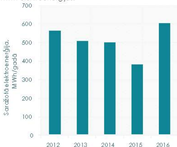
2.11. ATTĒLS: Rundāles novadā vietēji saražotie elektroenerģijas apjomi
