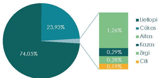
2.4. ATTĒLS: Biogāzes ražošanas potenciāla sadalījums novada teritorijā
