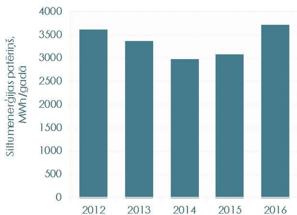
2.17.ATTĒLS: Kopējais siltumenerģijas patēriņš pakalpojumu un rūpniecības sektorā, ēkām, kas pieslēgtas Dobeles CSS
