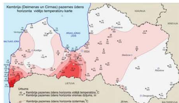
2.6. ATTĒLS: Kambrija pazemes ūdens horizonta vidējo temperatūru karte (Avots: LVĢMC)
