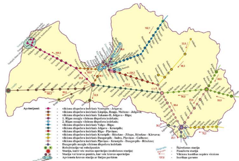
1.42.attēls. Latvijas dzelzceļa vilcienu kustības un kravas darba organizācijas shēma 2012. g.
